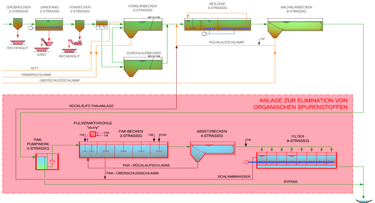
Abbildung 1: Fließschema PAK-Dosierung mit PAK-Rezirkulation und Rückführung PAK-Überschussschlamm in den Rücklaufschlamm der Biologie.
